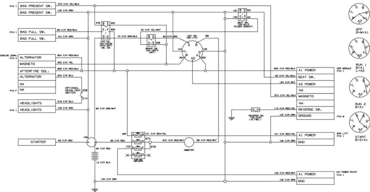
Schaltplan / Diagram
