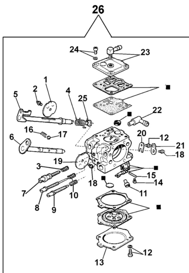
27 ■ KIT RIPARAZIONE REPAIR KIT
